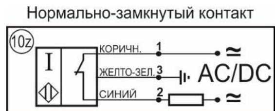
Схема соединения
