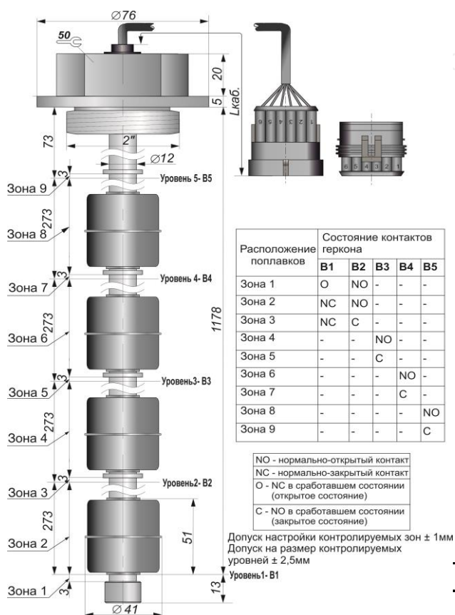
Габаритный чертеж
