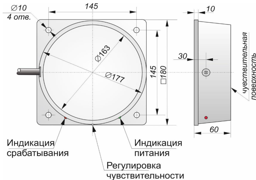
Габаритный чертеж
