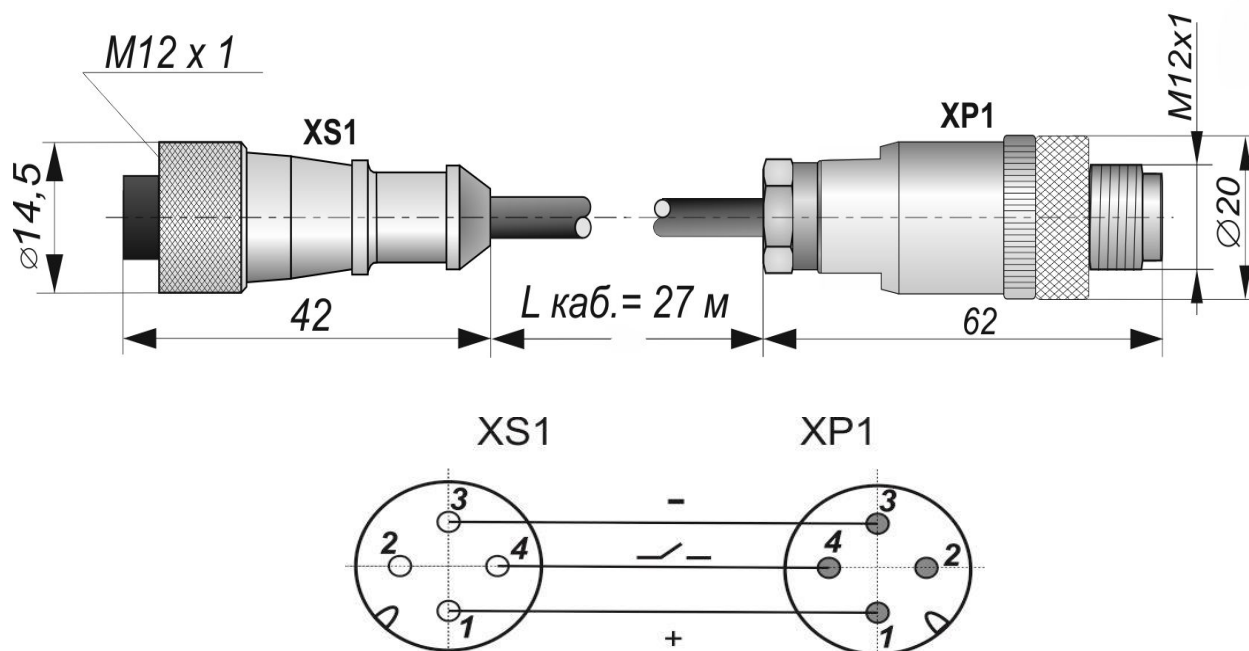
Габаритный чертеж
