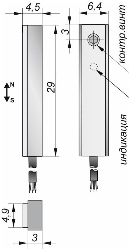
Габаритный чертеж
