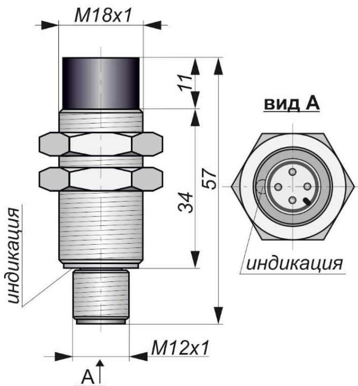
Габаритный чертеж
