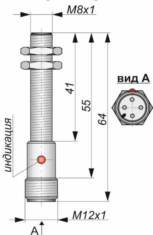
Габаритный чертеж
