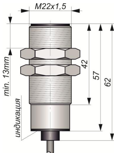
Габаритный чертеж
