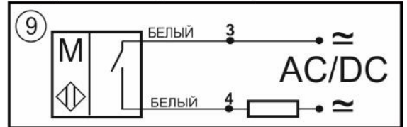
Схема соединения
