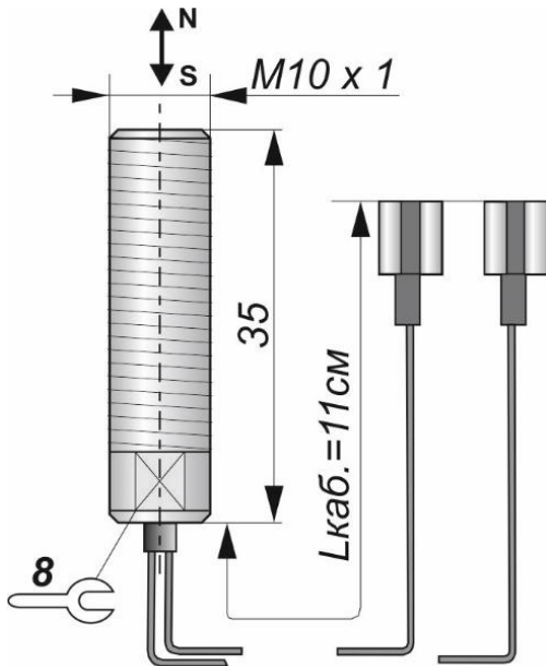
Габаритный чертёж
