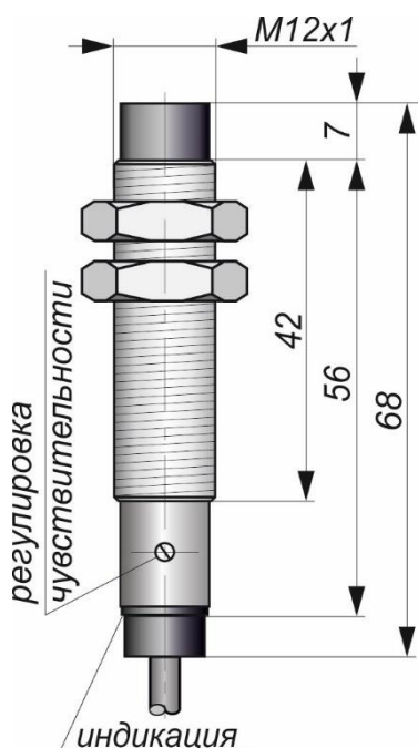
Габаритный чертеж
