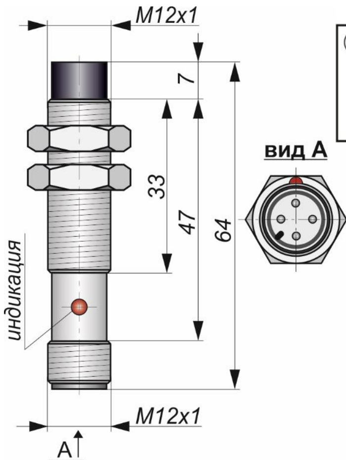
Габаритный чертеж
